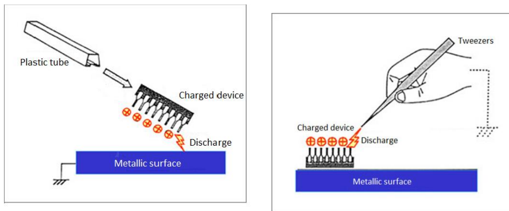
Fig 2.4 discharges IC
