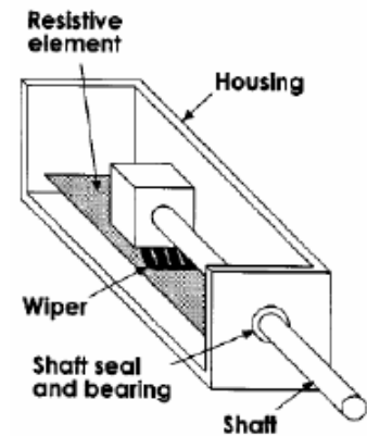
Potentiometer
