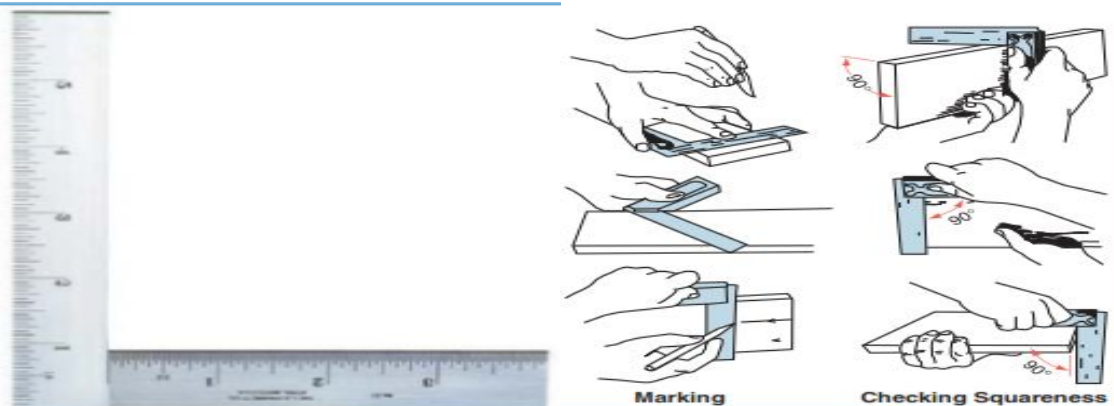
Fig. 3.10. Try square
