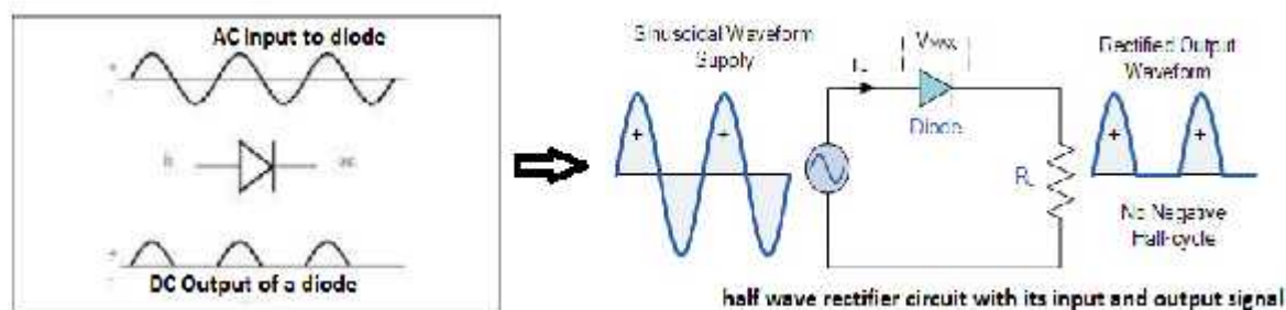
Fig. 3.26 Half wave rectifier
