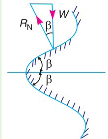
Fig. 10.14. V-thread.
