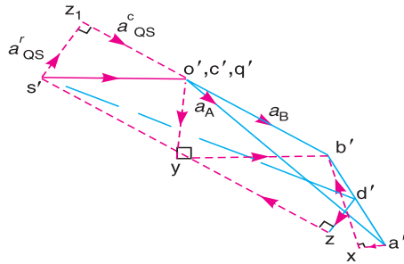
(d) Acceleration diagram.
