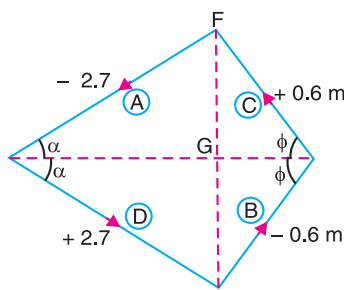
(d) Primary couple polygon.
