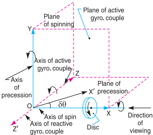
Fig. 14.2. Gyroscopic couple.
