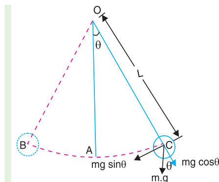
Fig 4.3. Simple pendulum.
