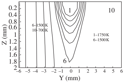
b) Isotherms
