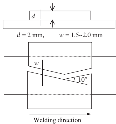
10.17 I-butt weld
