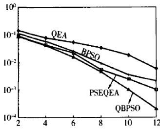
Fig. 2. The comparison of bit error rate (BER)
